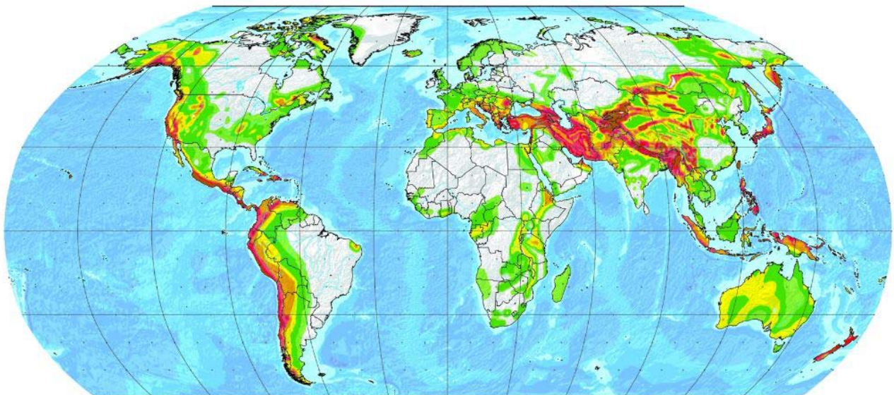
Fig. 1 Mappa mondiale delle zone sismiche
