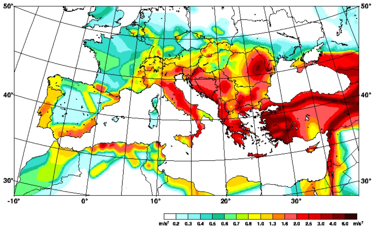
Fig. 2 Mappa delle zone sismiche nell'area del Mediterraneo
